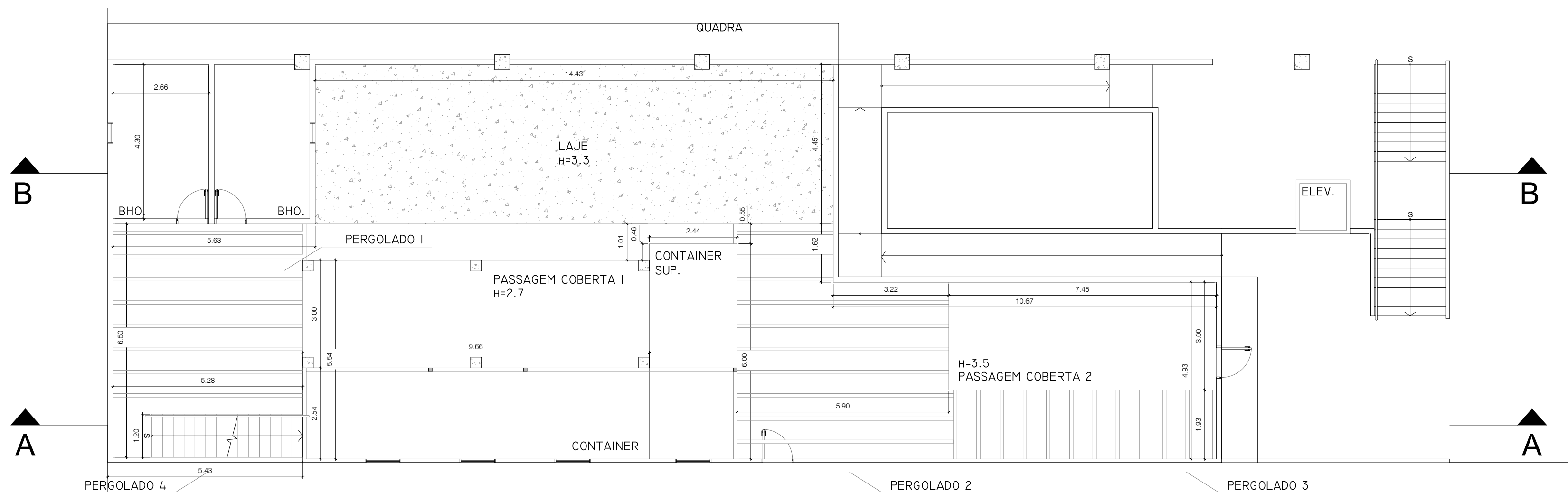
PLANTA 1 PAVIMENTO ESC 1:100
