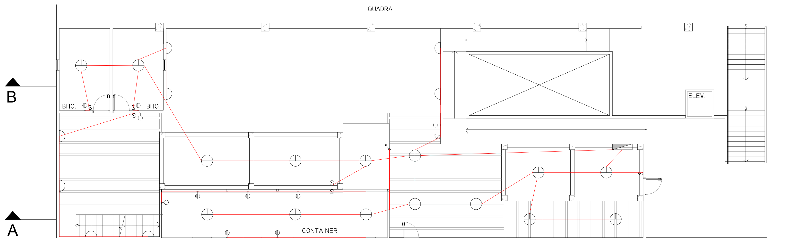
PLANTA TÉRREO ESC 1:100
