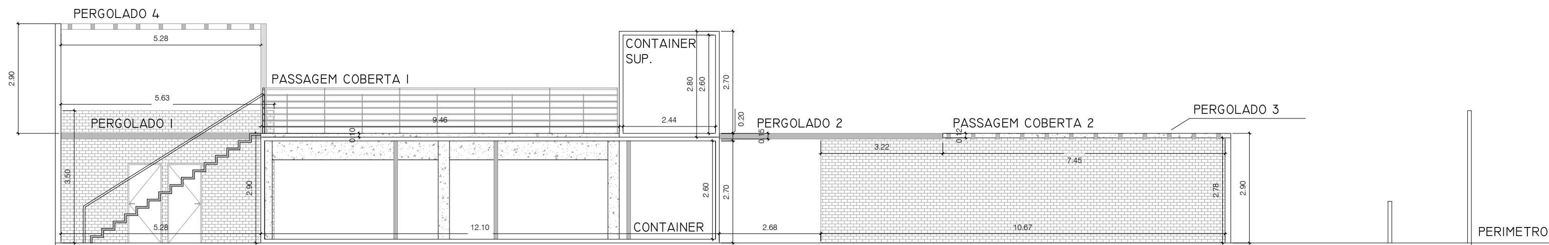
CORTE AA ESC: 1/100
